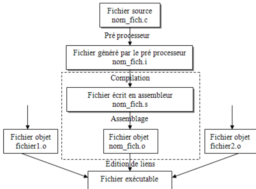
FIG. 1.1 – Étapes de création d'un exécutable à partir d'un code écrit en C
