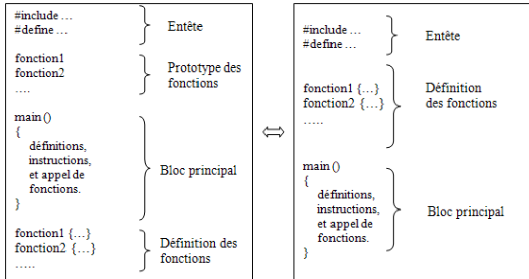
FIG. 2.1 – Structure d'un programme C
